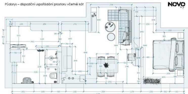
Půdorys – dispoziční uspořádání prostoru včetně kót
